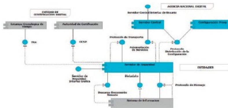
Ilustración 11. Arquitectura de Componentes (Fuente: Suministrada por la Agencia Nacional Digital)
